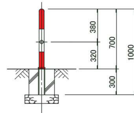
組立図
