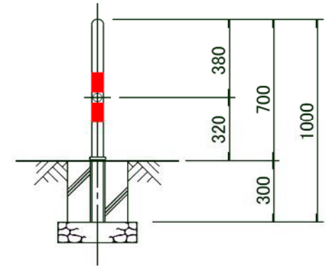
組立図
