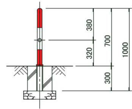
組立図
