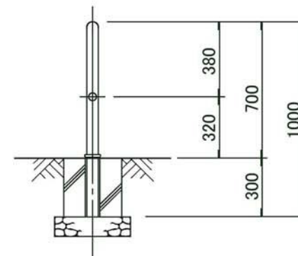
組立図
